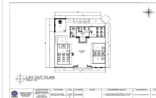
Gambar 4. Gambar 2D Kantor desa seraya
