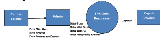
Gambar 4. Diagram Konteks
