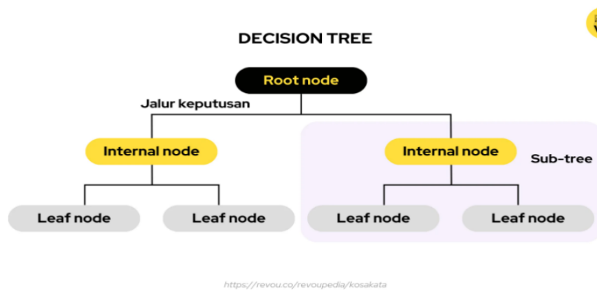
Gambar 2. Pohon Keputusan
